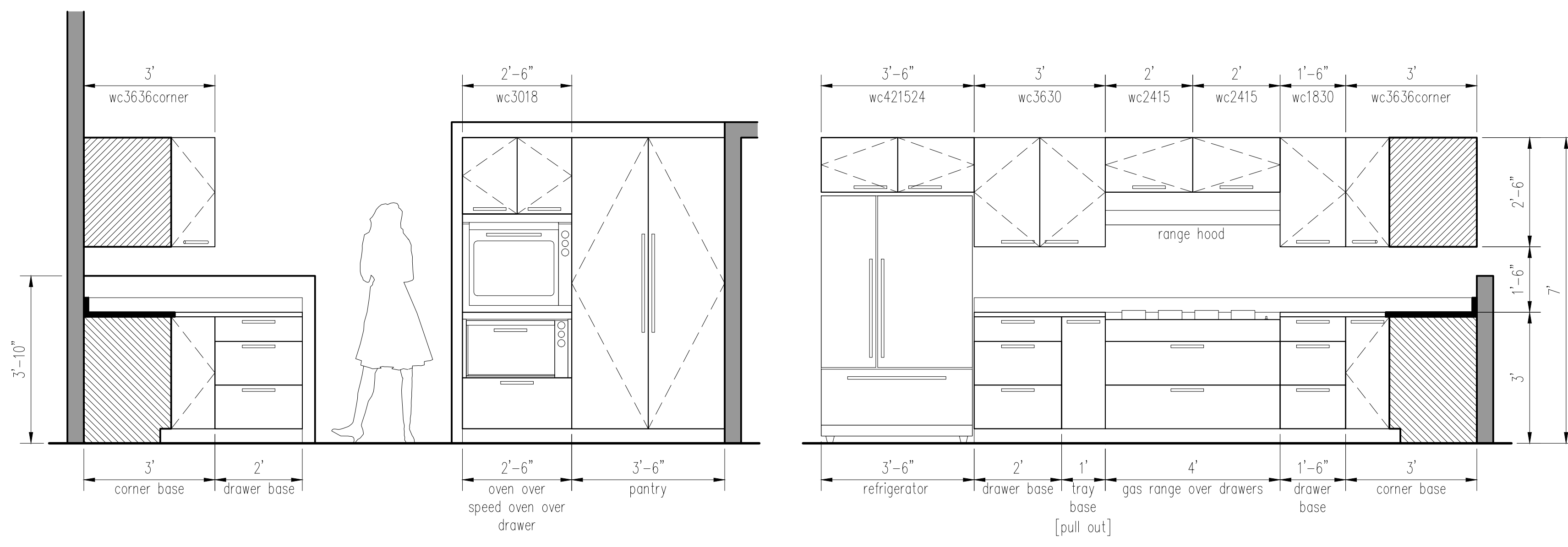
elevation A
